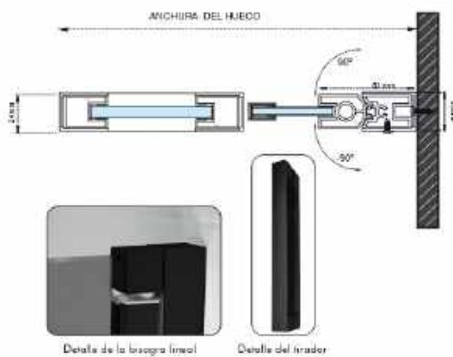
Sección del conjunto
