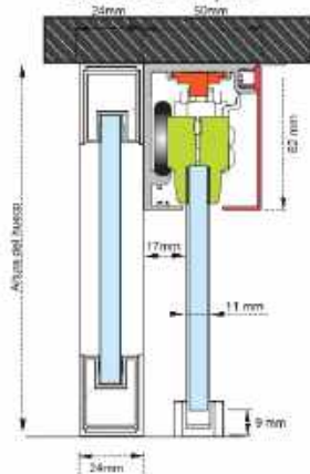
Detalle guío
