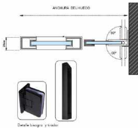
Sección del conjunto
